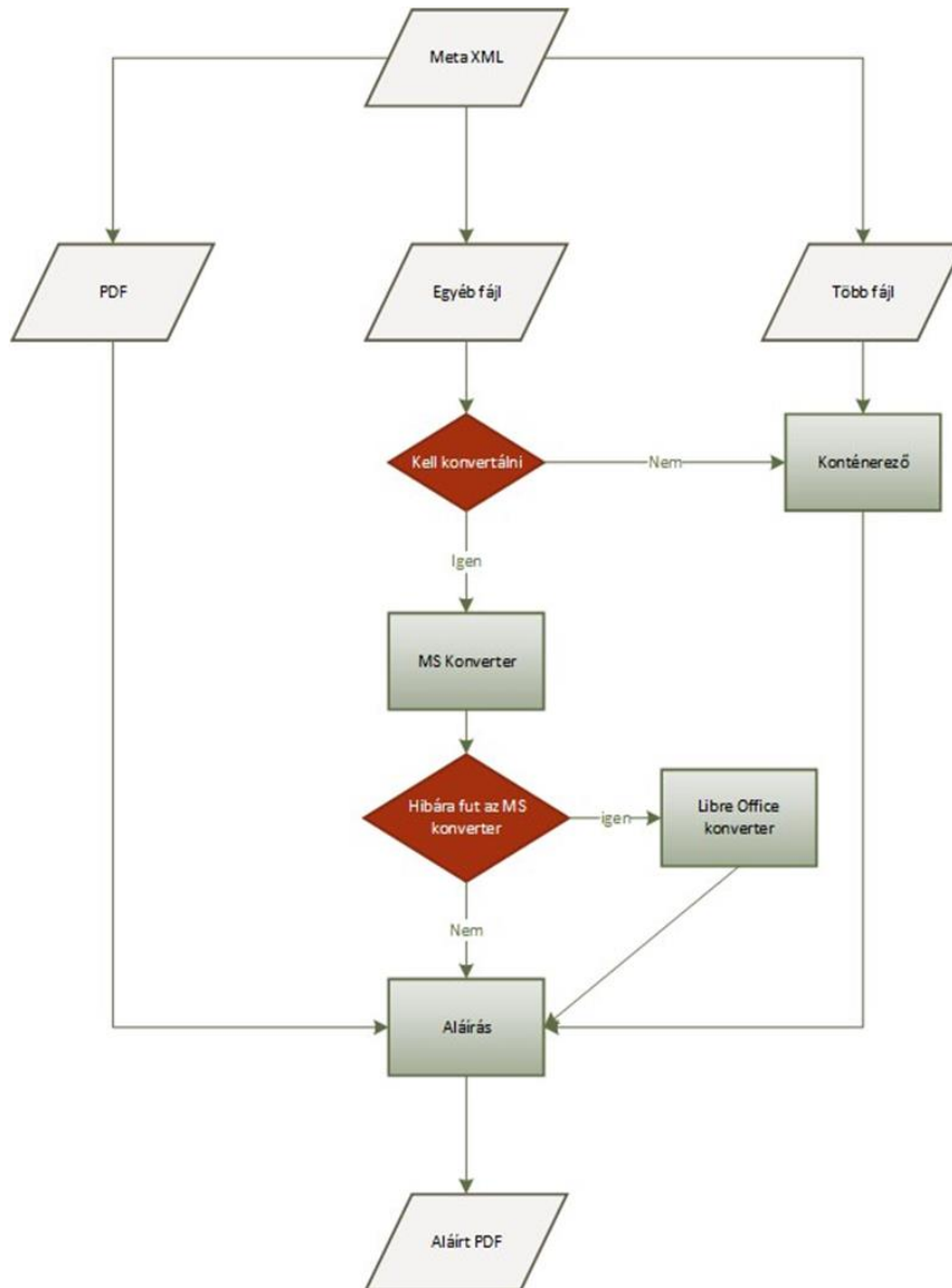
2. ábra: Az RZS Signer rendszerszintű működése
