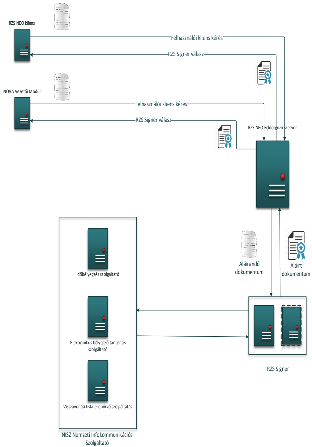
2.ábra: Az RZS Signer hitelesítés funkció rendszerszintű működése
